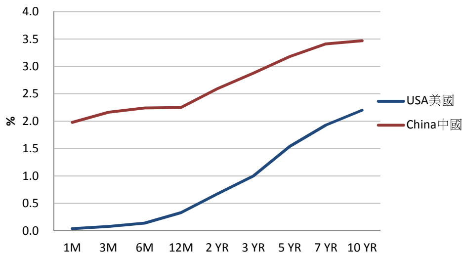
圖 1: 收益率曲線
